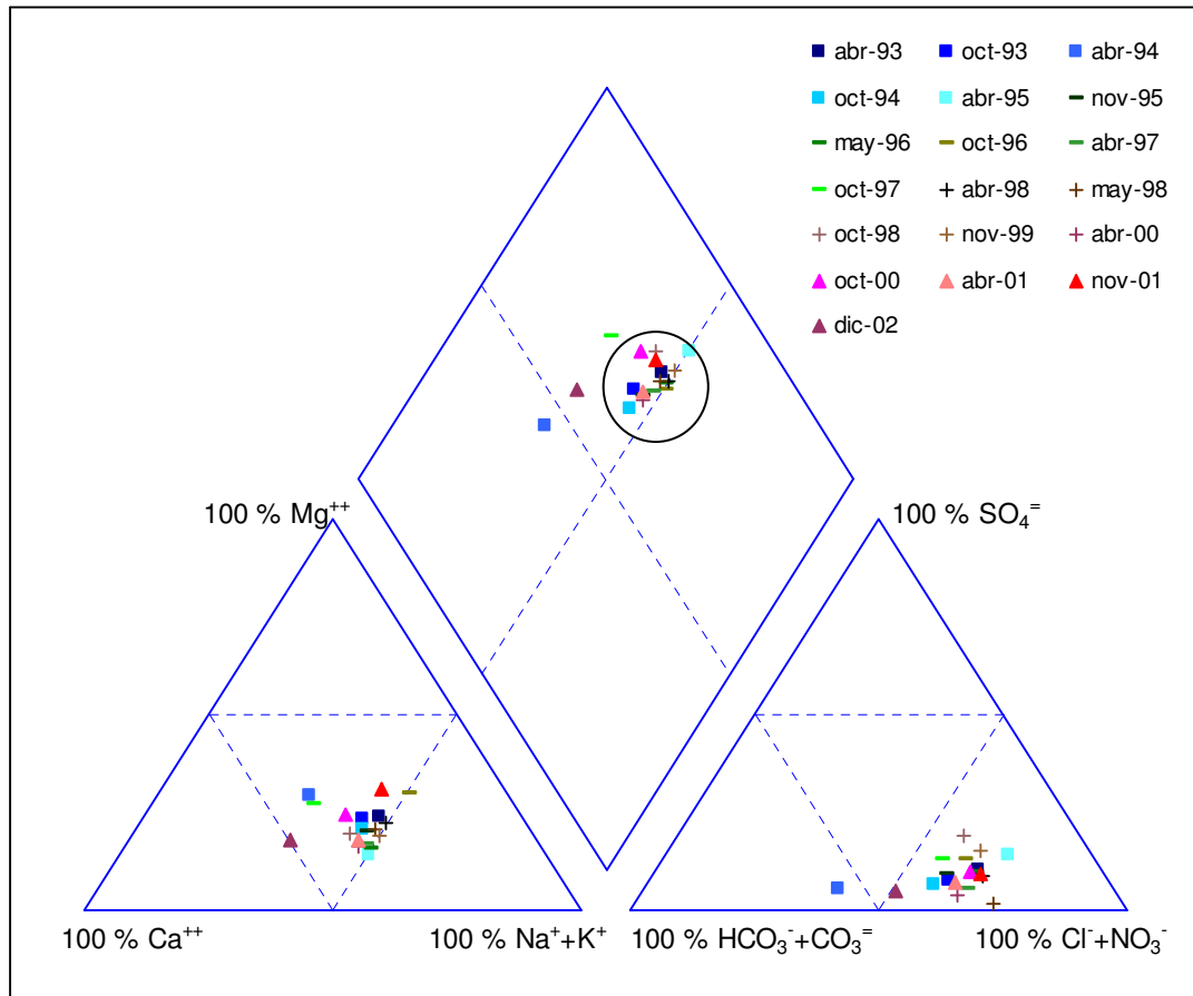
Fig. 3 Diagrama de Piper-Hill-Langelier de la captación nº 114210049.
