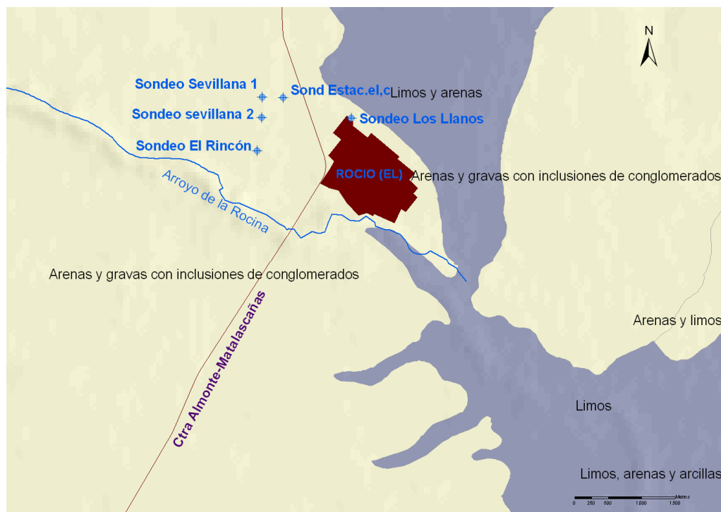
Fig. 1 Geología de la zona.
